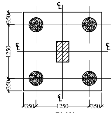
PLAN P.C. - 4 ( 4 - PILE ) 400 DIA. PILES
