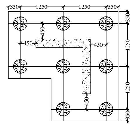
PLAN P.C. - 8 ( 8 - PILE ) 400 DIA. PILES
