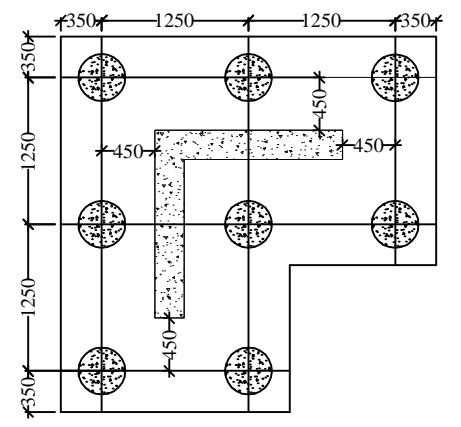
PLAN P.C. - 8 ( 8 - PILE ) 400 DIA. PILES
