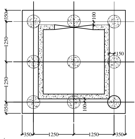
PLAN P.C. - 9 ( 9 - PILE ) 400 DIA. PILES
