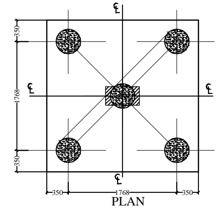
PLAN P.C. - 5 ( 5 - PILE ) 400 DIA. PILES
